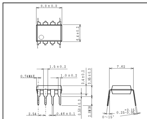
DIP-8
