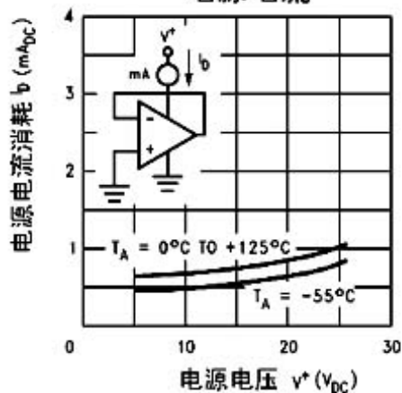
电源电流
