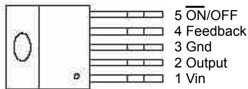
TO220B-5L/TO220-5L
