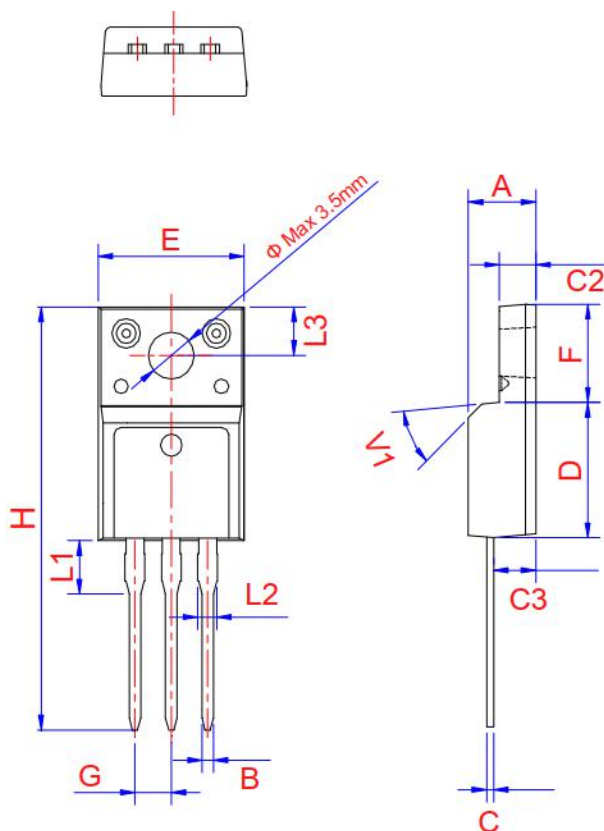
TO-220F Ins
