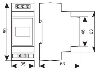
Габаритные размеры
