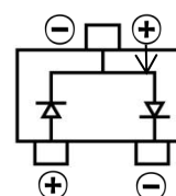
BAT54S:KL4
