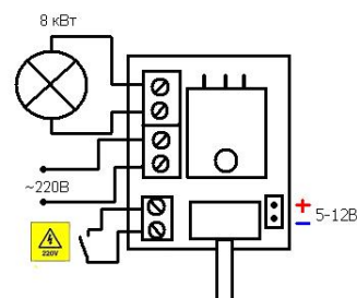
Схема подключения. Рис. 2
