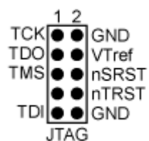
Распиновка JTAG разъема
