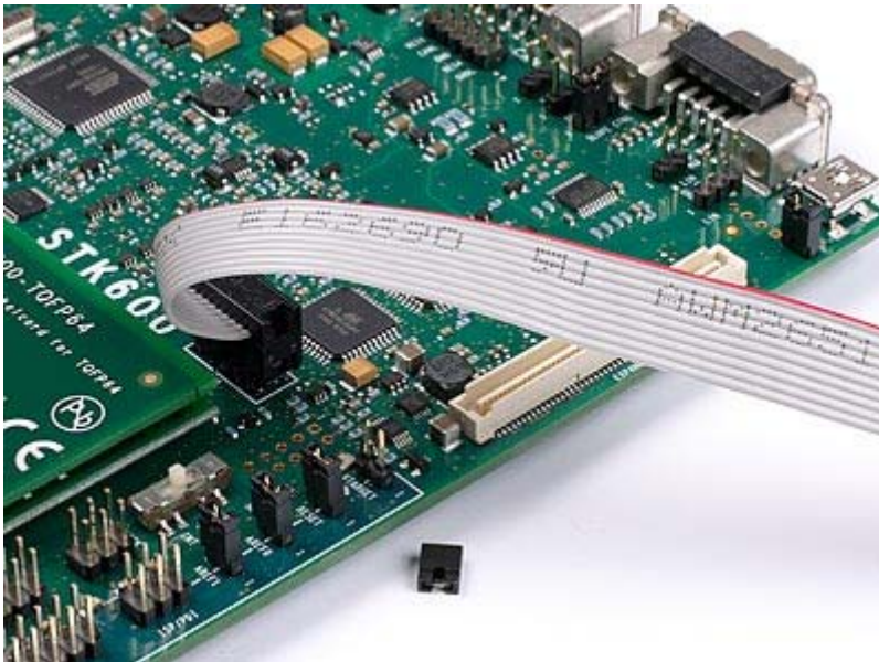
ISP программирования внешней системы, используя 10-контактный разъем
