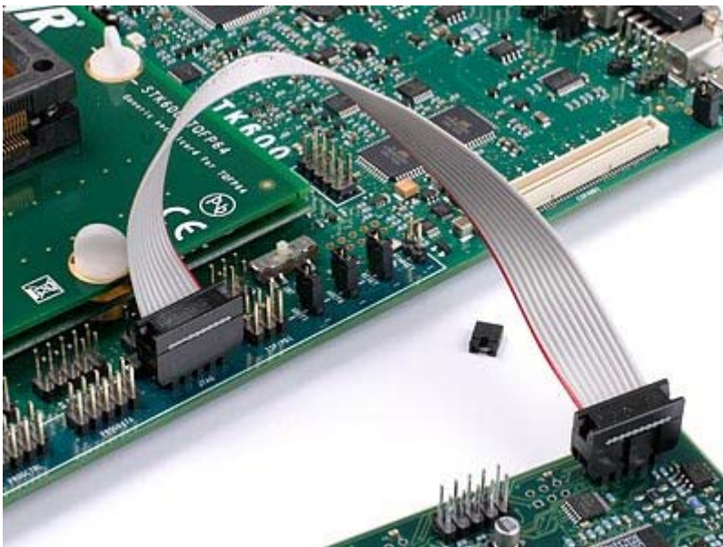
JTAG программирование внешней системы
