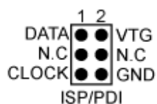
Распиновка PDI разъема
