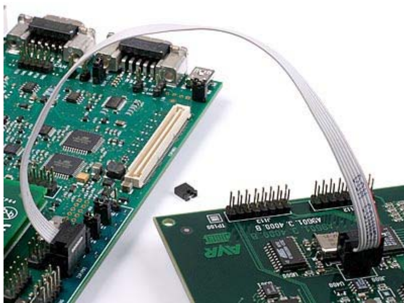
ISP или PDI программирование внешней системы с помощью 6-контактного разъема
