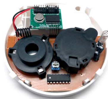
Вид устройства изнутри. Рис. 2
