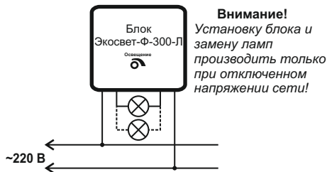
Рис.1. Схема монтажа
