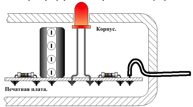
Рис.5 Установка светодиода на печатной плате
